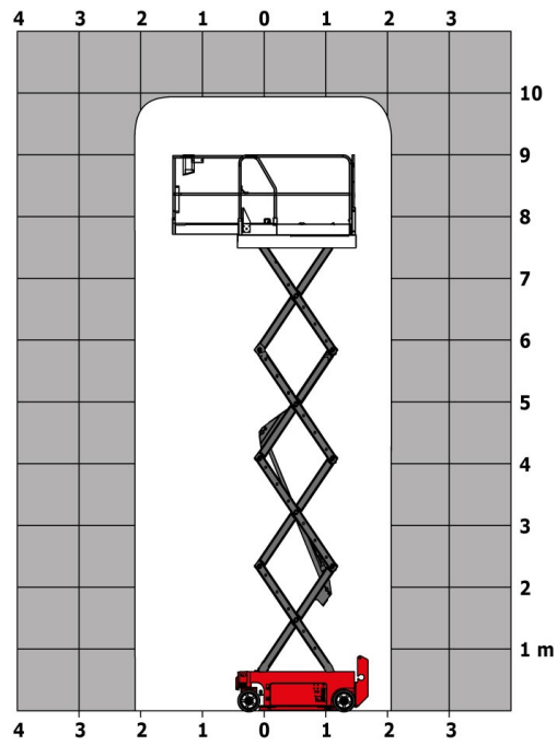
Lastdiagramm
